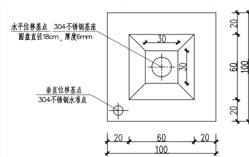
观测基点平面图
