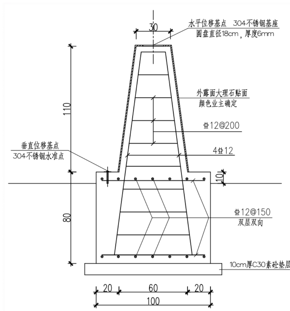
观测基点剖面图
