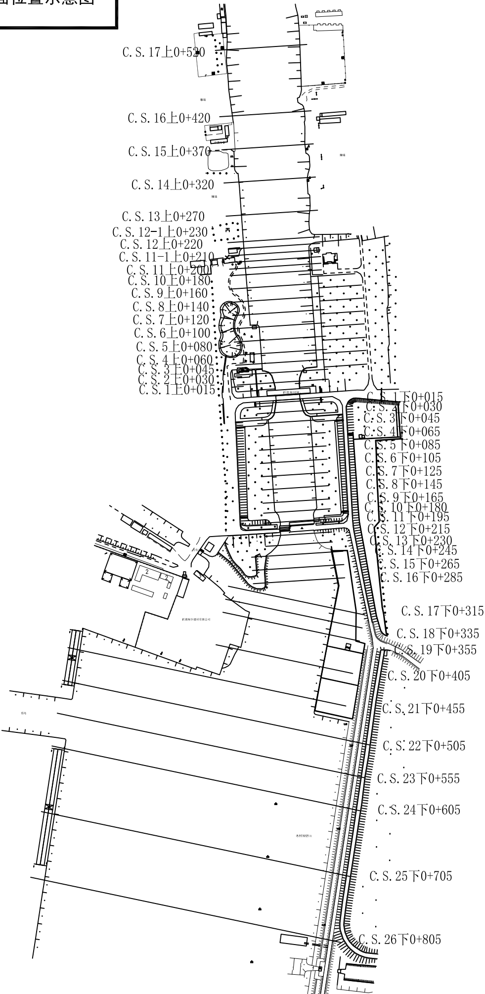
新江海河闸断面位置示意图
